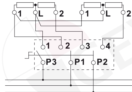
Kochplatte 2x3 Anschlüsse 1x3-poliger Viertaktschalter
