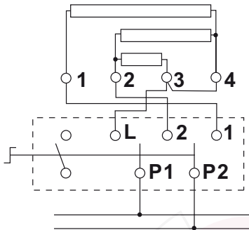
Kochplatte 4 Anschlüsse 2-poliger Fünftaktschalter
