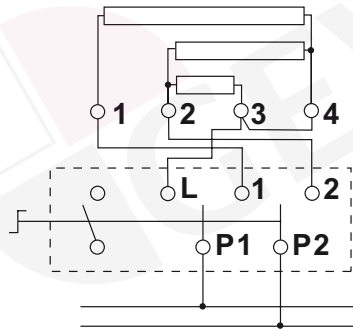
Kochplatte 4 Anschlüsse 2-poliger Viertaktschalter
