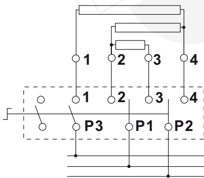
Kochplatte 2x3 Anschlüsse 2x2-poliger Viertaktschalter
