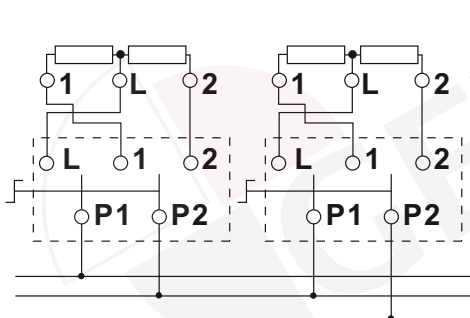
Kochplatte 2x3 Anschlüsse 2x2-poliger Viertaktschalter
